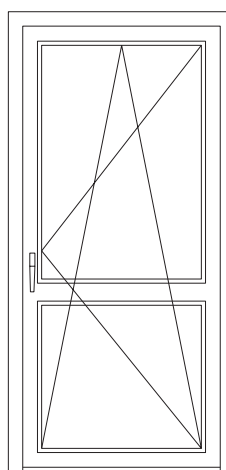
✓ vrata bez barijera zaokretno-otklopna
