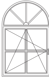
✓ ◆ Polukružni prozor zaokretno-otklopni sa prečkama/fiksni nadsvjetlom
