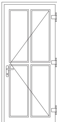
✓ kućna vrata 1-kril. sa otvaranjem prema unutra i prečkama
