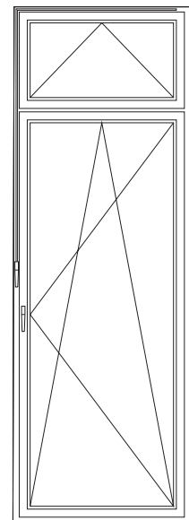
✓ zaokretno-otklopna vrata sa otklopnim nadsvjetlom
