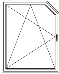
✓ zaokretno-otklopni prozor sa kosinom
