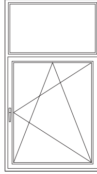
✓ zaokretno-otklopni prozor sa fiksnim nadsvetlom
