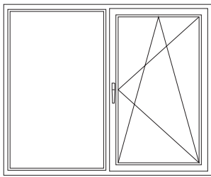
✓ dvodijelni prozor fiksni/zaokretno-otklopni
