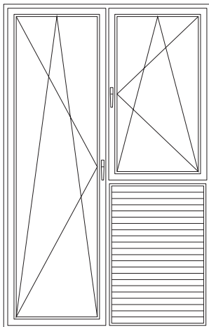
✓ prozor sa balkonskim vratima, zaokretno-otklopna vrata i zaokretno-otklopni prozor sa parapetom
