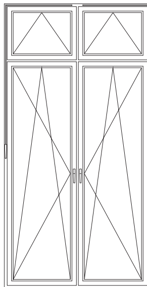
✓ dvodijelna vrata zaokretno-otklopna/zaokretno-otklopna sa otklopnim nadsvjetlom
