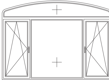
✓ ◆ Lučni prozor sa nadsvjetlom zaokretno-otklopni/fiksni/zaokretno-otklopni
