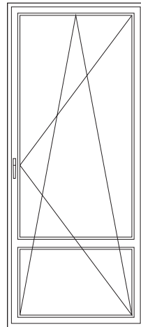
✓ zaokretno-otklopna vrata sa prečkom u krilu
